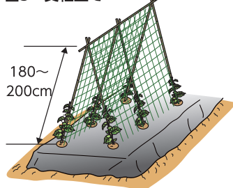
図3 支柱立て
